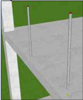
1 - Mise en place du potelet
